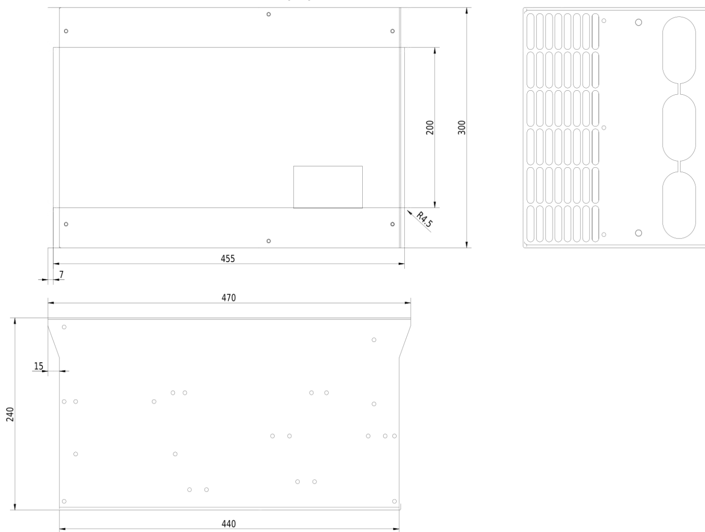
Rozmerový výkres V900 - 55kW 4T0550
