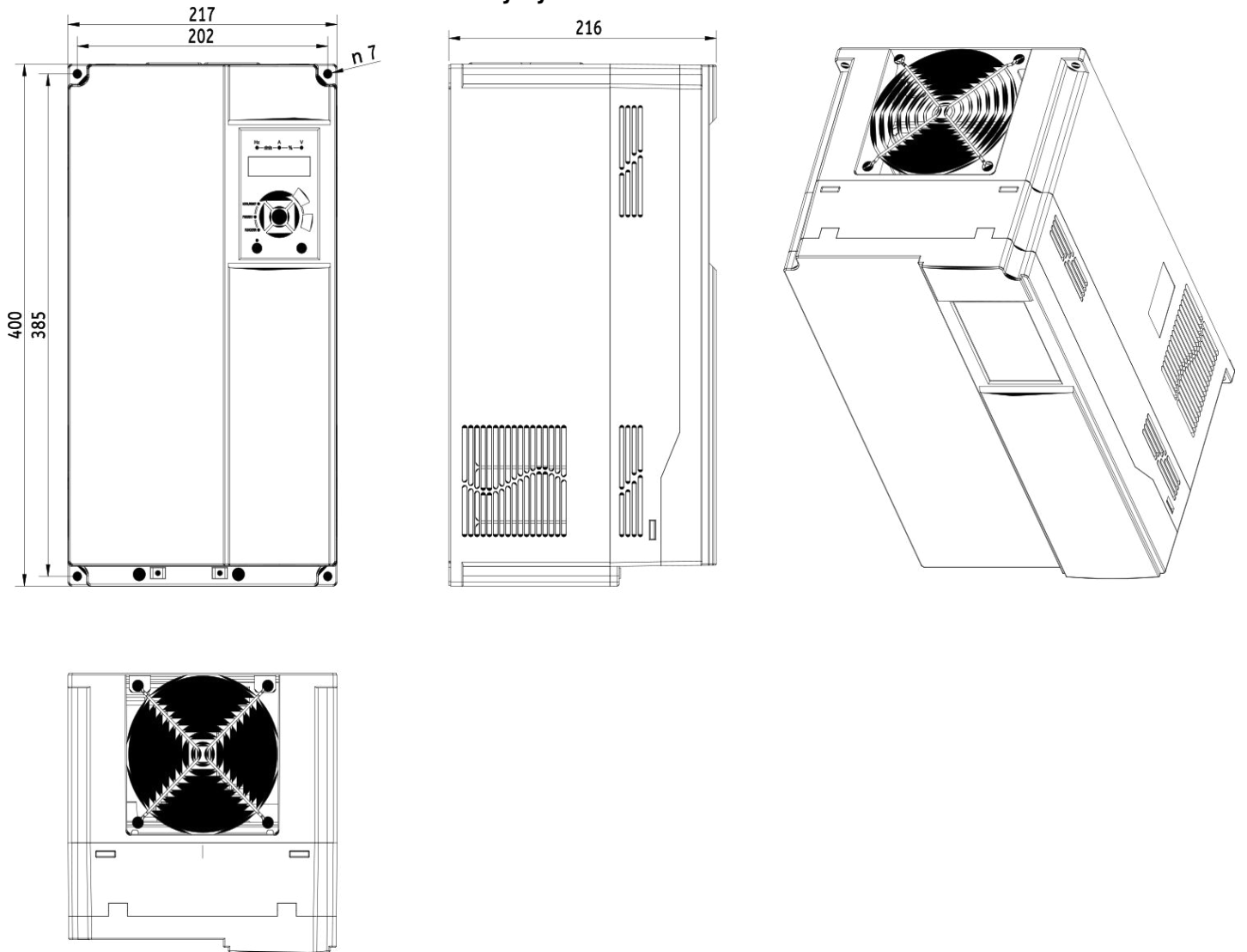
Rozmerový výkres V900 - 37kW 4T0370
