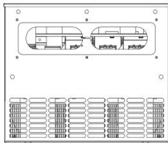
Rozmerový výkres V810 - 160kW 4T1600
