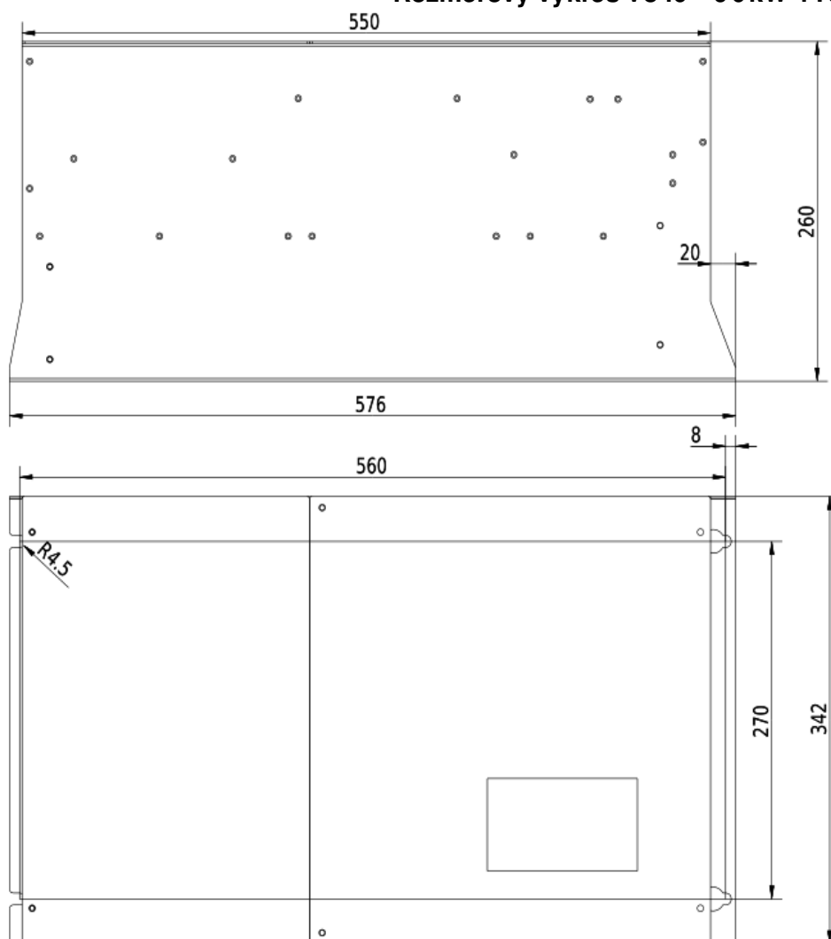
Rozmerový výkres V810 - 90kW 4T0900
