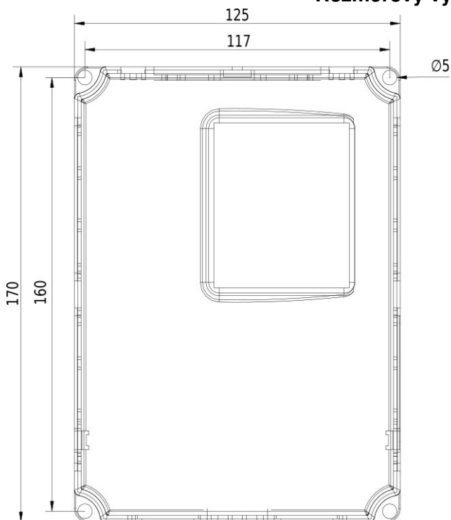
Rozmerový výkres V810 - 2,2kW 4T0022
