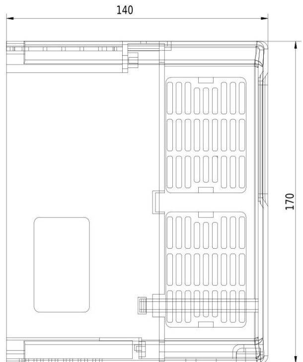
Rozmerový výkres V810 - 0,75kW 4T0007
