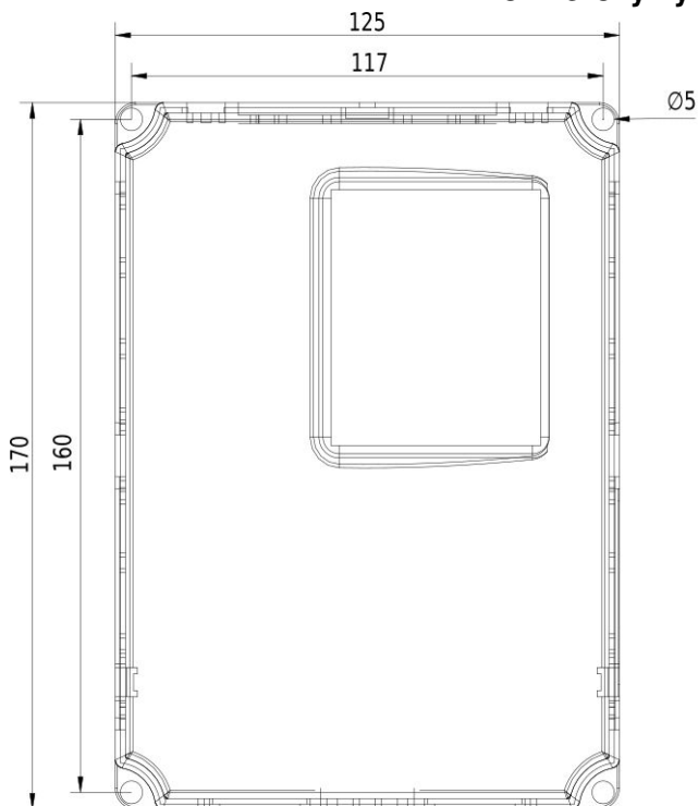
Rozmerový výkres V810 - 0,75kW 4T0007
