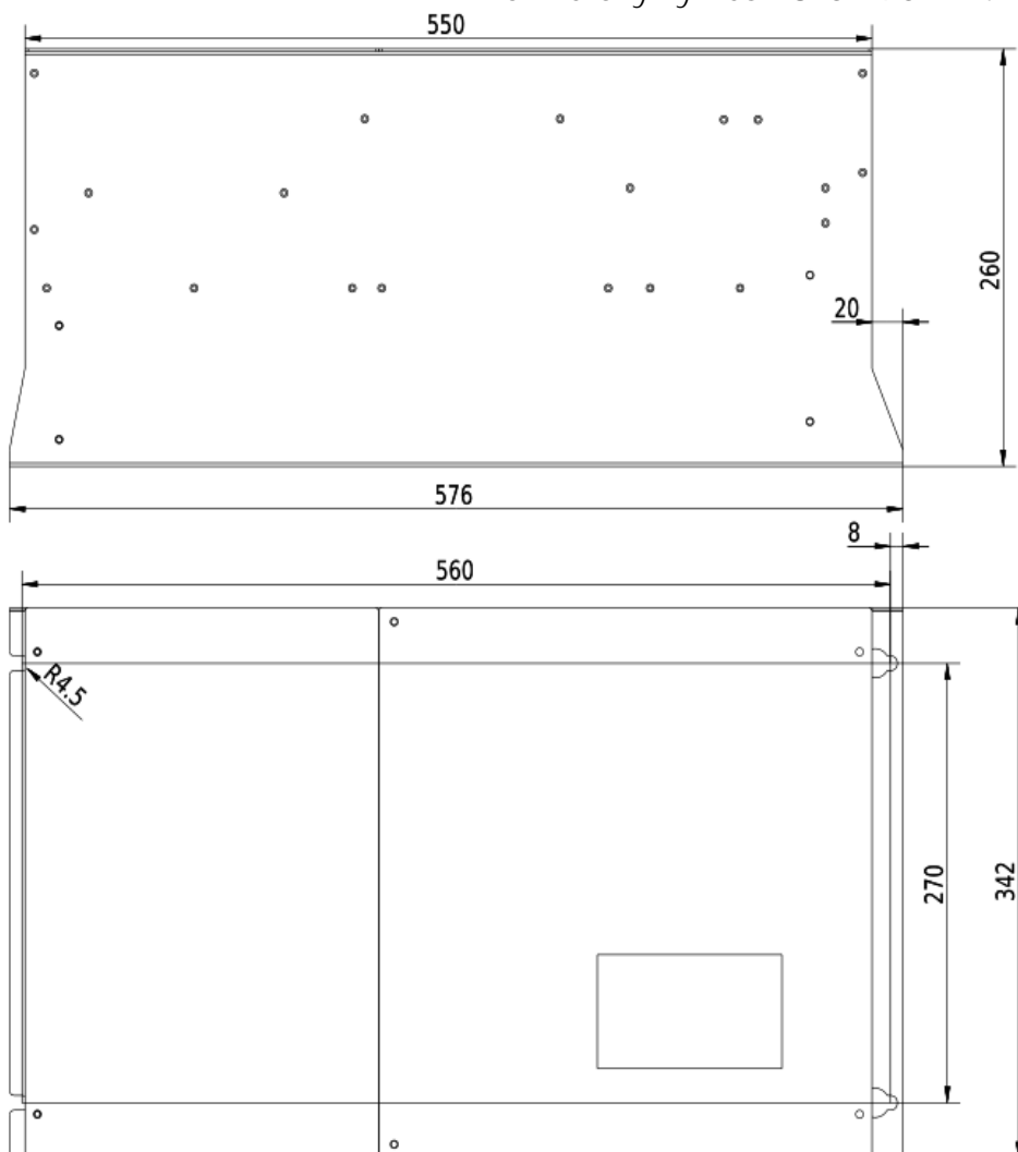
Rozmerový výkres V810 - 90kW 4T0900
