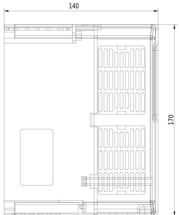
Rozmerový výkres V810 - 0,4kW 4T0004
