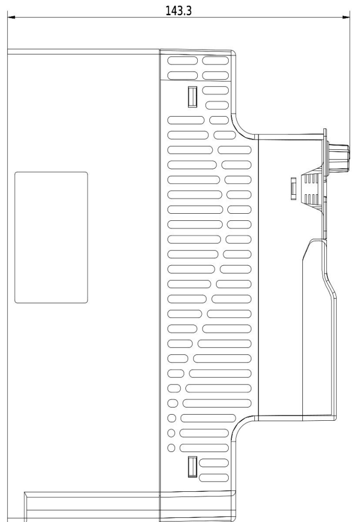
Rozmerový výkres V800 - 3kW 4T0030
