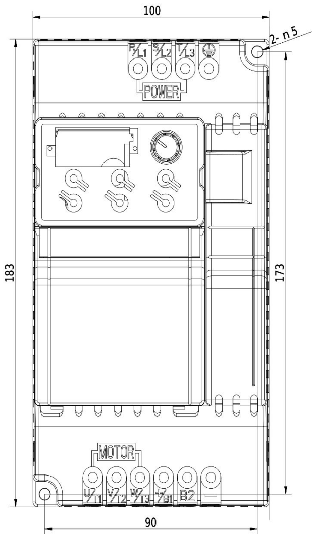
Rozmerový výkres V800 - 3kW 4T0030
