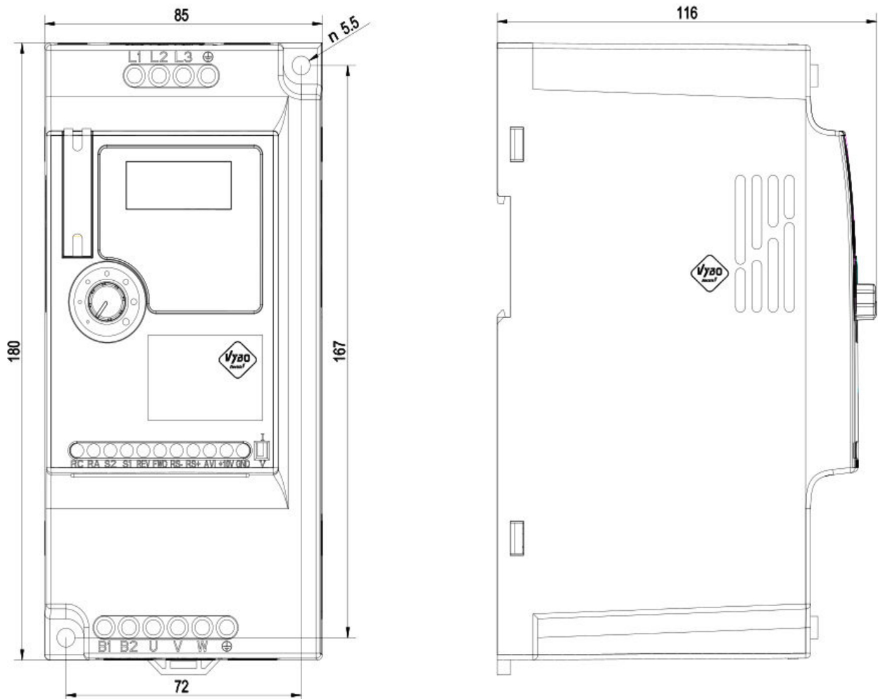
Rozmerový výkres A550 PLUS - 5,5kW 4T0055
