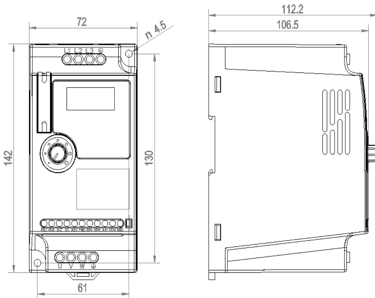
Rozmerový výkres A550 PLUS - 2,2kW 4T0022
