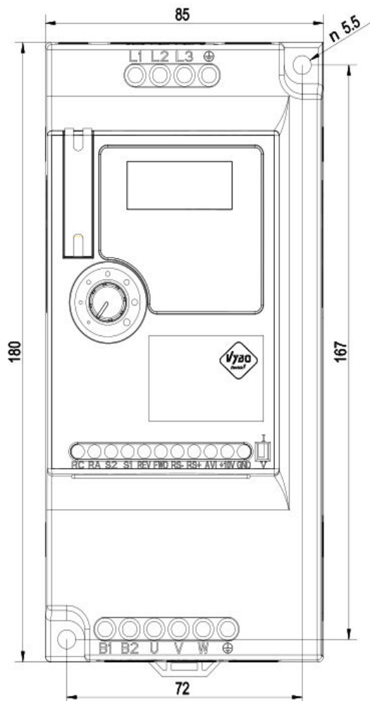
Rozmerový výkres A550 PLUS - 3kW 2S0030
