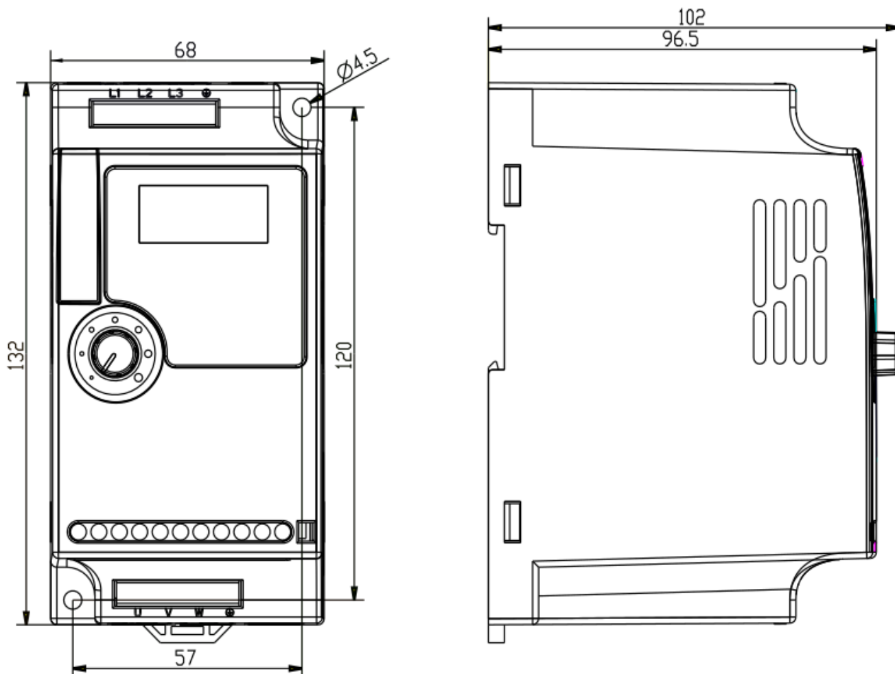
Rozmerový výkres A550 PLUS - 0,75kW 2S0007
