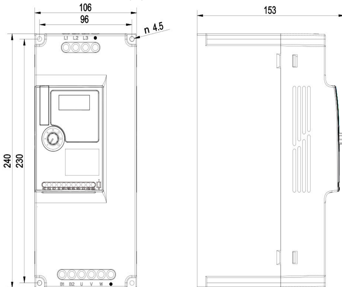
Rozmerový výkres A550 PLUS - 11kW 4T0110
