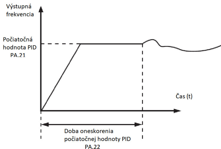
Obrázok 4-25 Funkcie počiatočnej hodnoty PID
