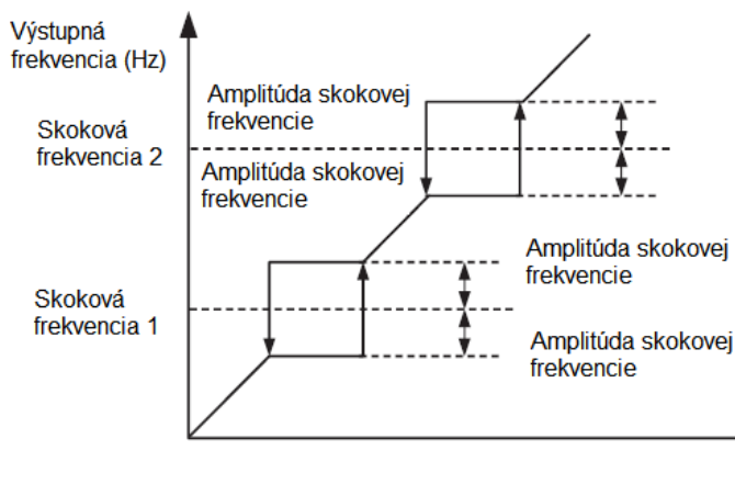
Obrázok 4-12: Princíp skokových frekvencií a amplitúdy
