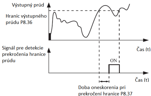
Obrázok 4-20 Detekcia prúdu
