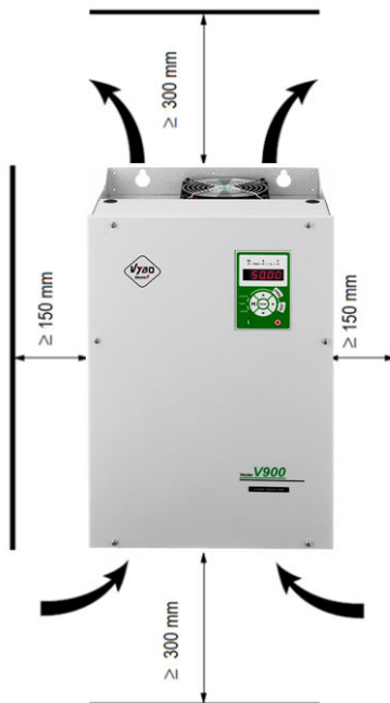
Umiestnenie meničov veľkosti C1,C2,C3
