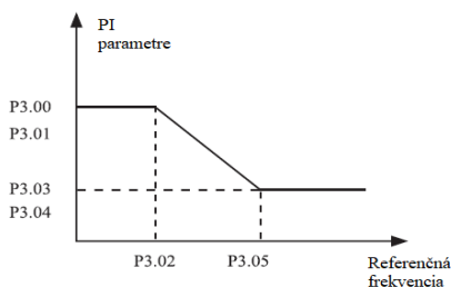
Obrázok 4-4: Vztah medzi frekvenciou chodu a parametrami PI
